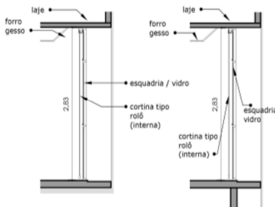
Corte A.
