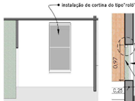
Vista Interna - Apoio ESC.: 1:100
