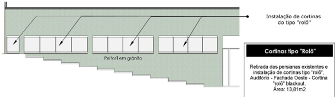
Vista Interna - Auditório ESC.: 1:100
