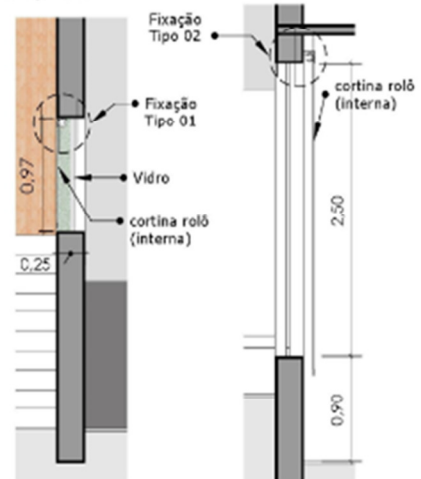
Corte A ESC.: 1:50
