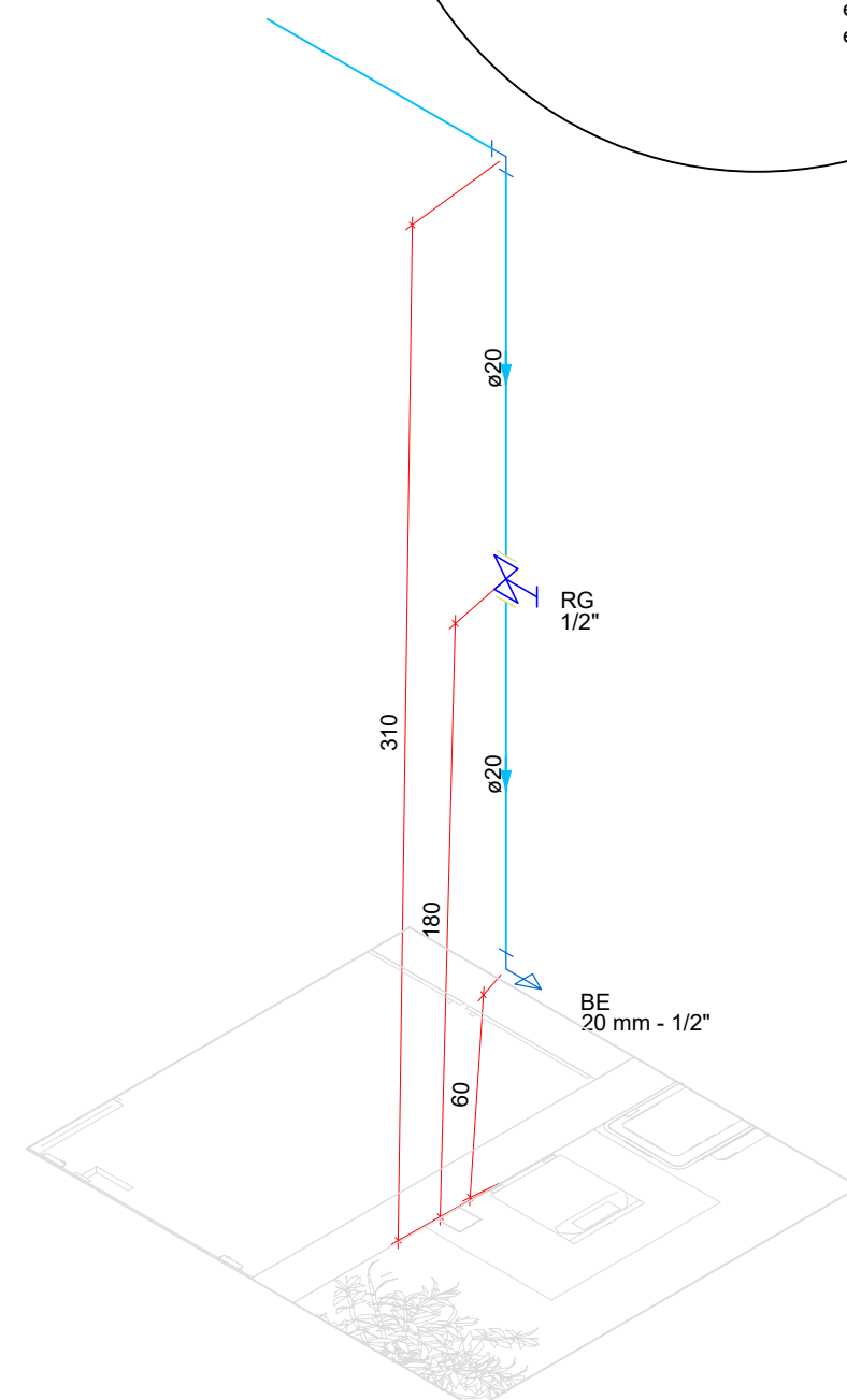
Detalhe HID-3 Escala 1:25
