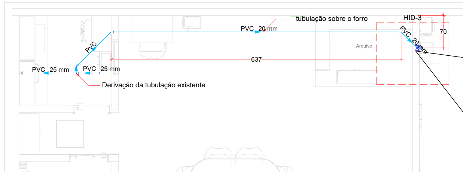
1 Planta Baixa Hidráulico ESCALA 1:50
