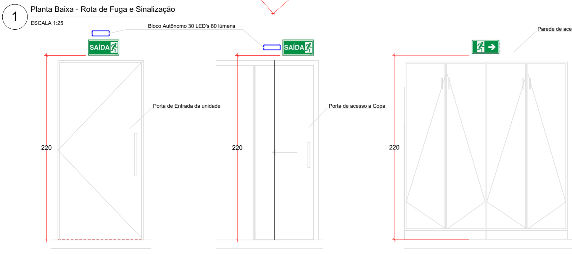
1 Planta Baixa - Rota de Fuga e Sinalização ESCALA 1:25
