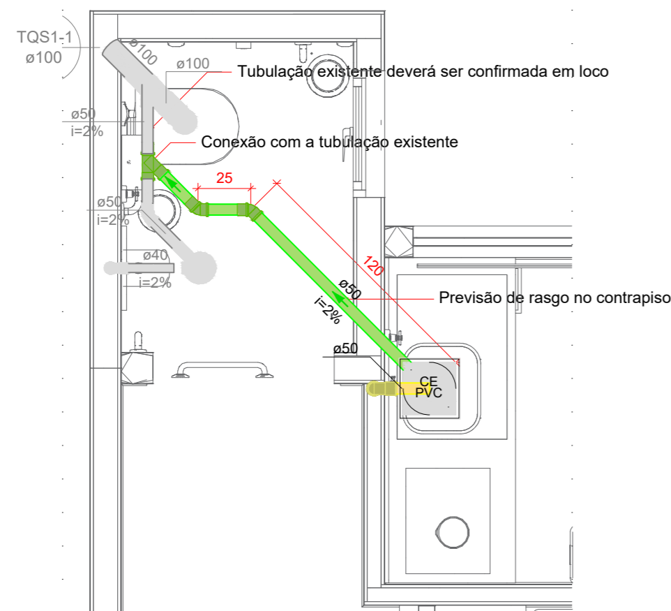
Detalhe SAN-1 Escala 1:25
