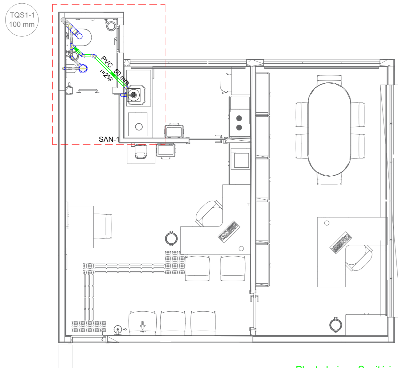
Planta baixa - Sanitário Escala 1:100
