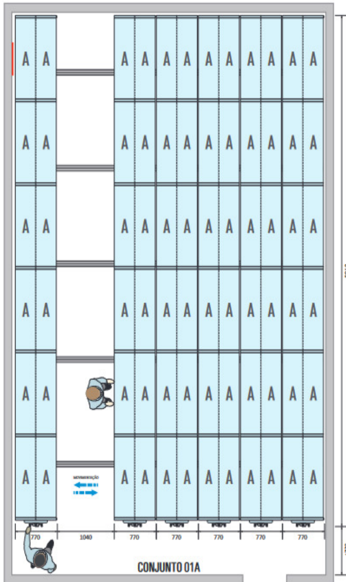
PLANTA BAIXA | ESCALA 1:60
