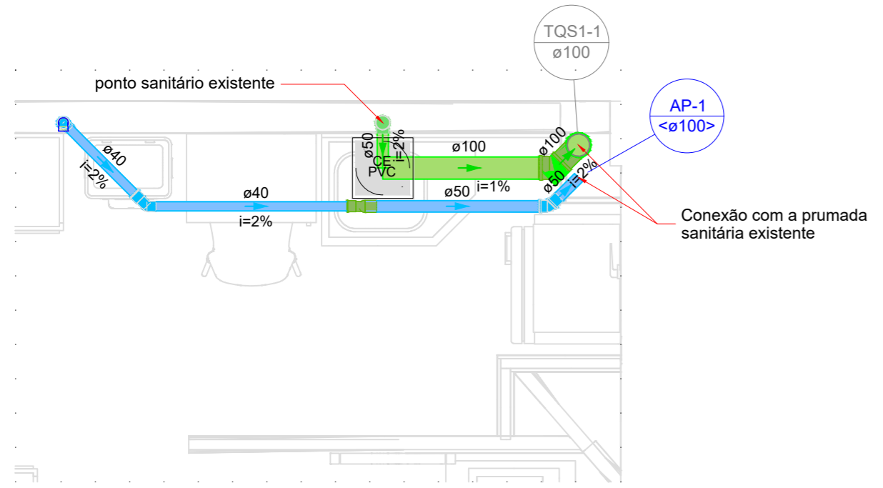
Detalhe SAN-1 Escala 1:25
