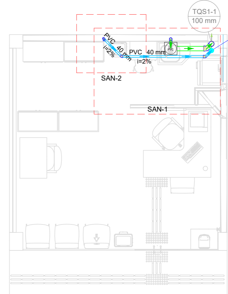
2 Planta Baixa - Sanitário ESCALA 1:50
