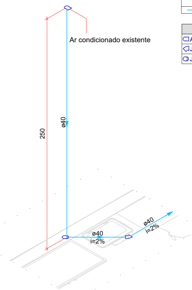
Detalhe SAN-2 Escala 1:25
