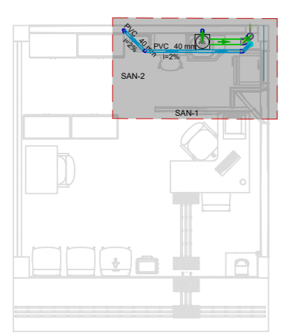
1 Planta Baixa - área de intervenção ESCALA 1:100
