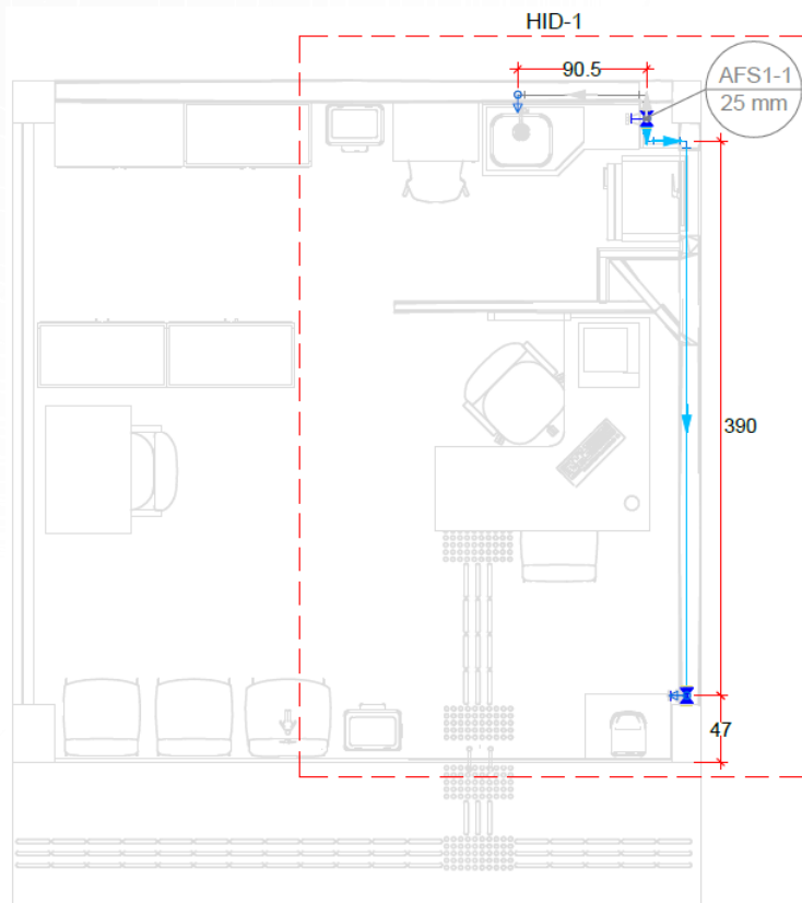
Planta baixa - Hidráulico
