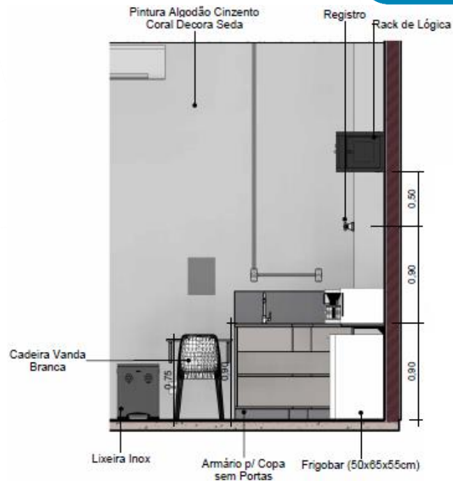
Corte A - Copa
