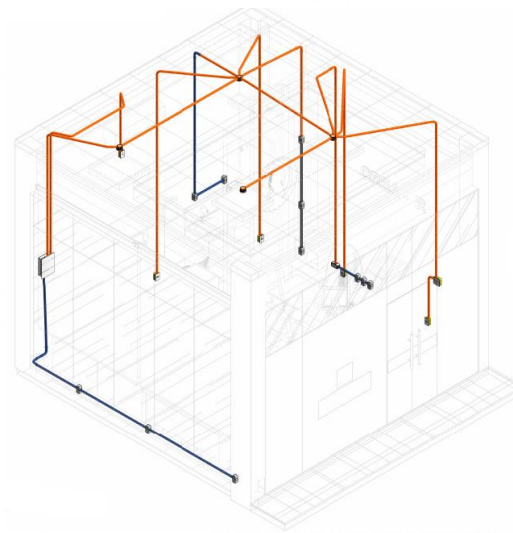
Vista 3D - Elétrico
