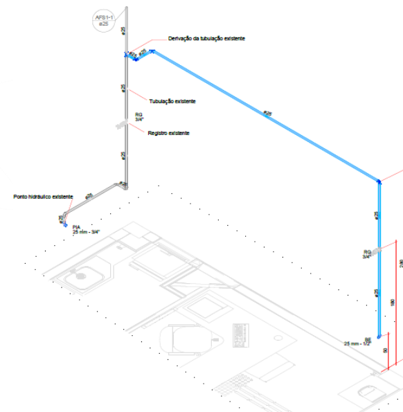
Detalhes das Instalações Hidráulicas
