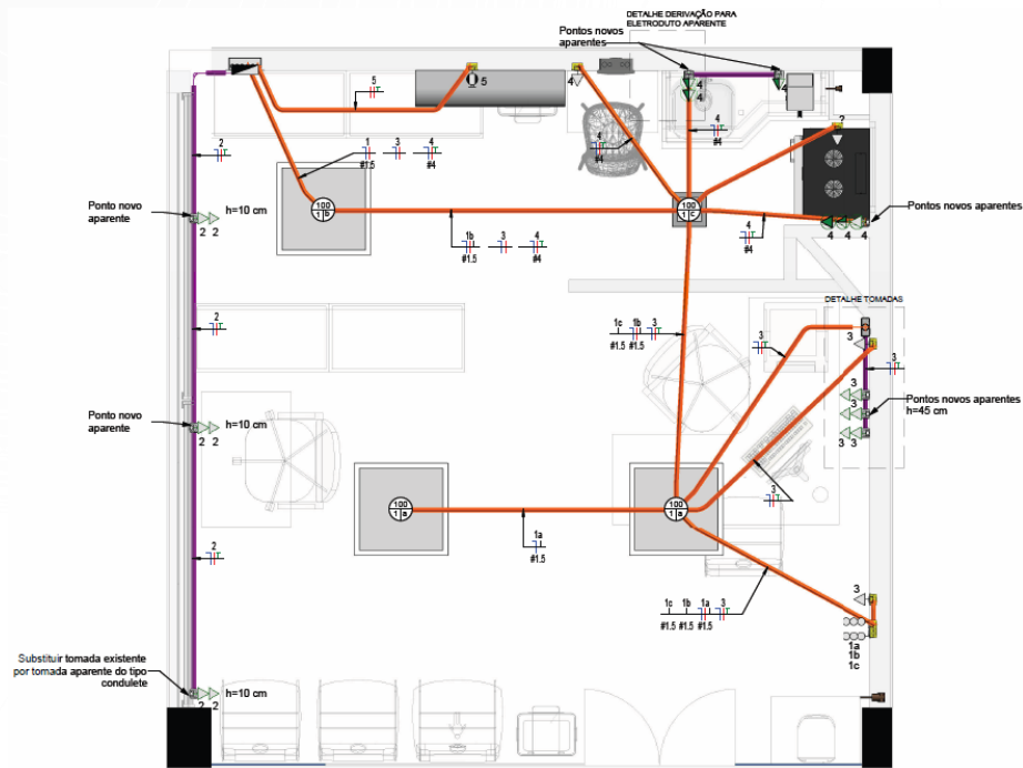
Planta baixa - Elétrico
