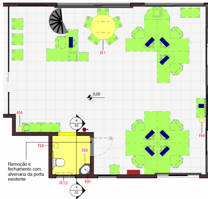
1 Térreo - Itens a Retirar 1:50
