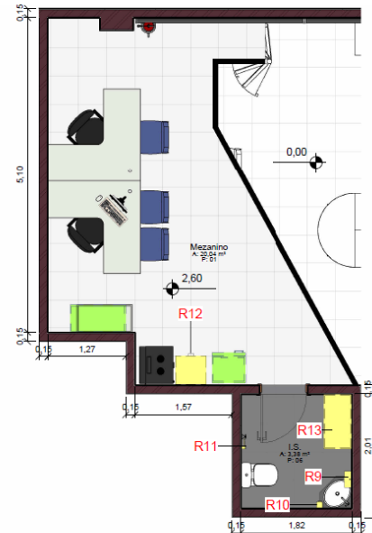
2 Mezanino - Itens a Retirar 1:50
