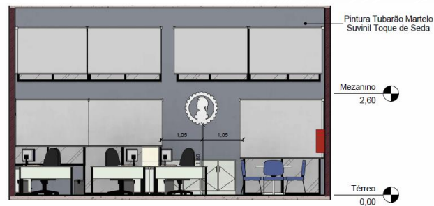
E Corte E 1 : 50
