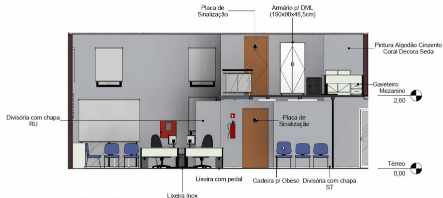
C Corte C 1 : 50
