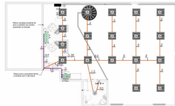
PLANTA BAIXA - MEZANINO
