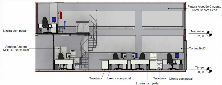
B Corte B 1 : 50
