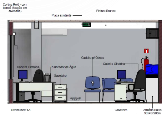
B Corte B 1 : 25
