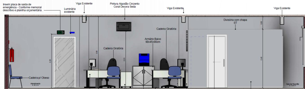
A Corte A 1 : 25
