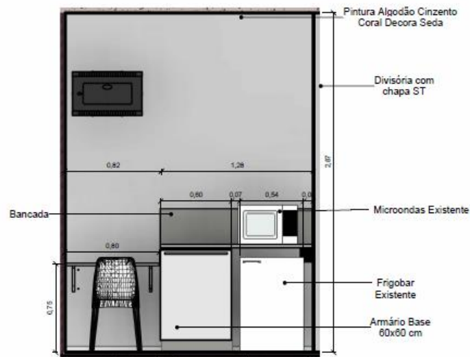
Corte copa
