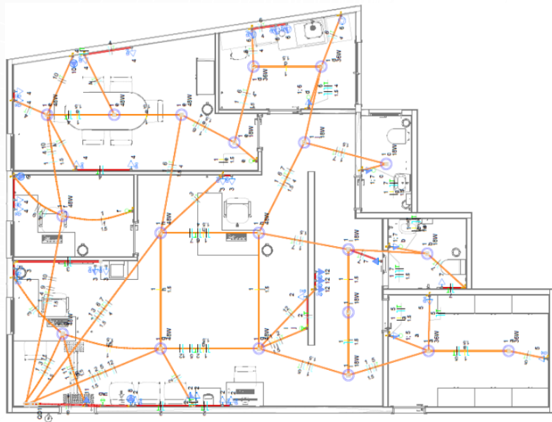
Planta baixa
