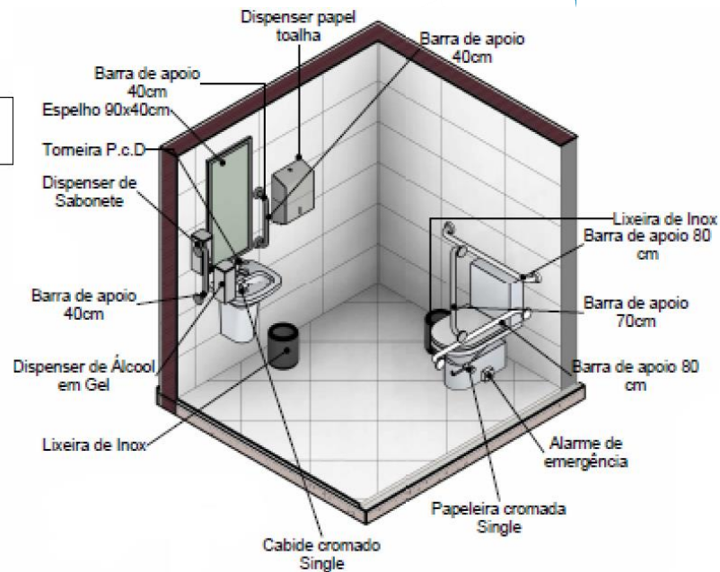
Instalações sanitárias
