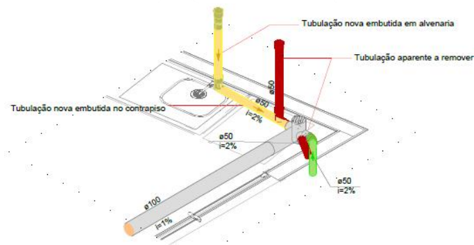
Detalhe isométrico
