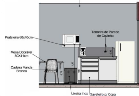
Corte copa
