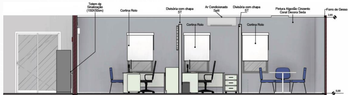
Corte C
