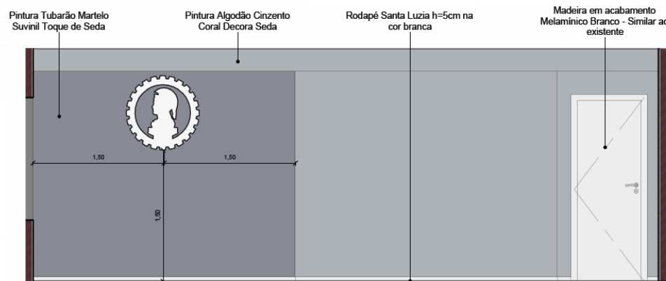
Detalhe revestimento
