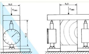
Figura 3 - Prensa para tensionar corpo prova. Fonte: ABNT (1997, p. 58).
